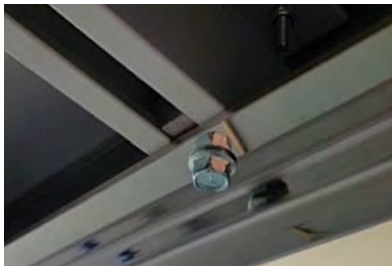
부식 방지용 알루미늄 소재 적용 (크로스 멤버 / 서브 프레임)
