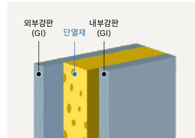
E-TRACK & BELT(하이 내장탑차) GI평판(40mm)
