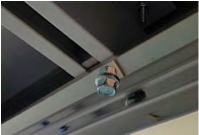
부식 방지용 알루미늄 소재 적용 (크로스 멤버 / 서브 프레임) 고강도 리어액슬 (허용하중 6.6톤)
