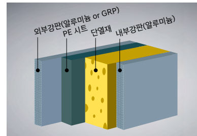
이트랙 & 벨트 판넬구조
