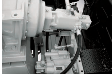
고성능 펌프 & 모터 (이튼)
