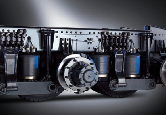
후축 에어 서스펜션 (4bag)
