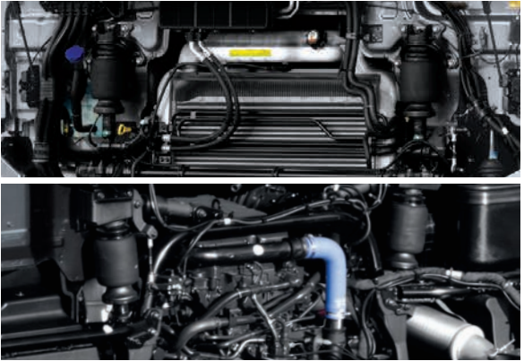
폴 플로팅 캡 에어 서스펜션 (전, 후)
