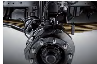
전축 멀티링크 서스펜션
