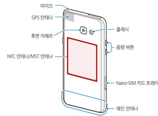
중앙 NFC 안테나 예시
