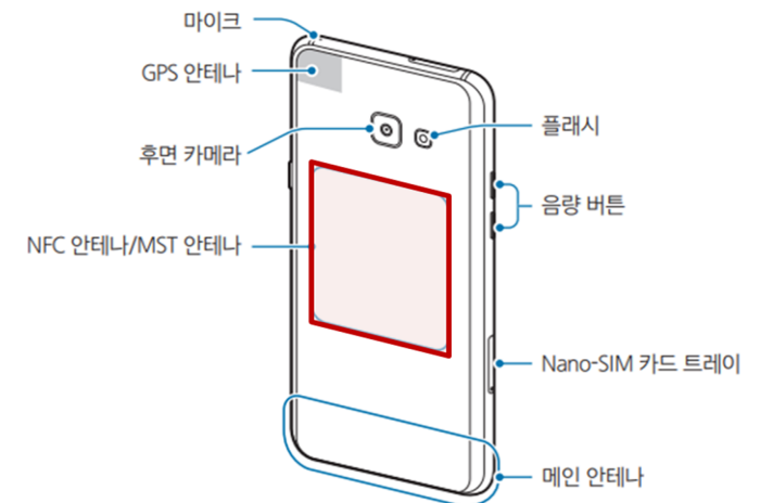
중앙 NFC 안테나 예시
