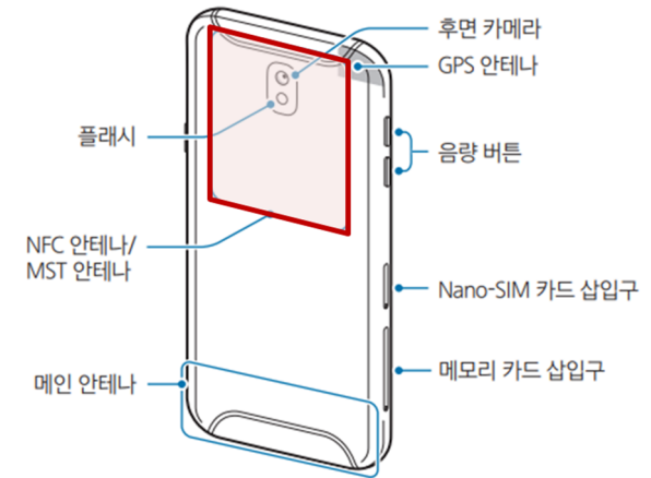
상단 NFC 안테나 예시
