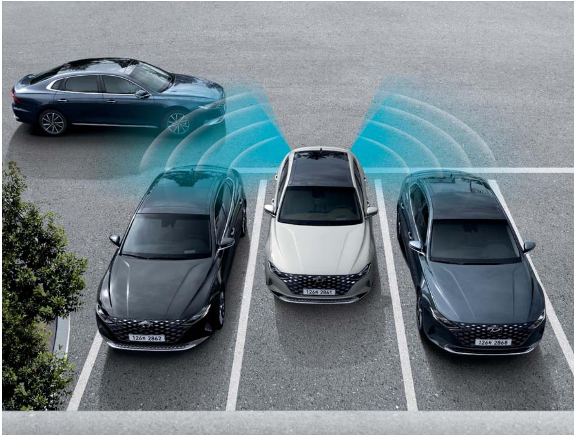
후방 교차 충돌방지 보조 후진 시 후측방 사각지대에서 접근하는 차량을 감지하여 운전자에게 경고해줍니다. 필요시 브레이크를 제어하여 후방 충돌을 방지할 수 있게 도와줍니다.
