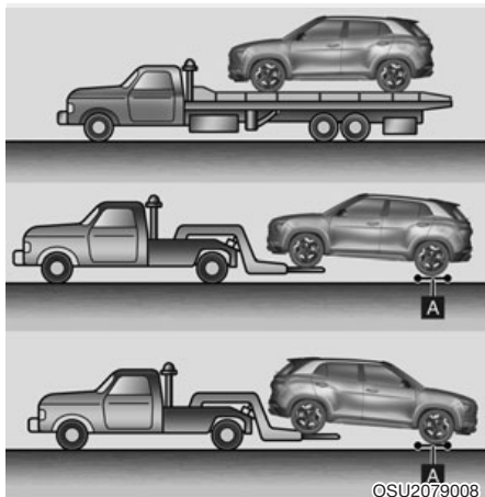
[А]: Буксировочная тележка
