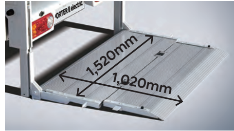
전동유압식 리프트 시스템 (허용하중 : 600kg)
