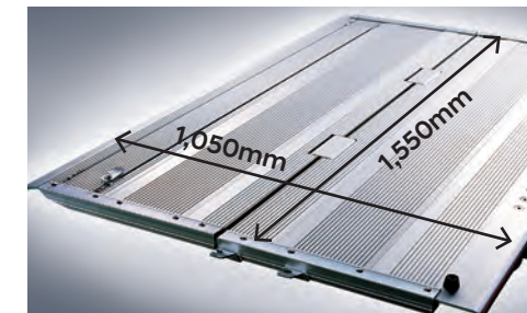
턴인타임 리프트 시스템 및 플레이트
