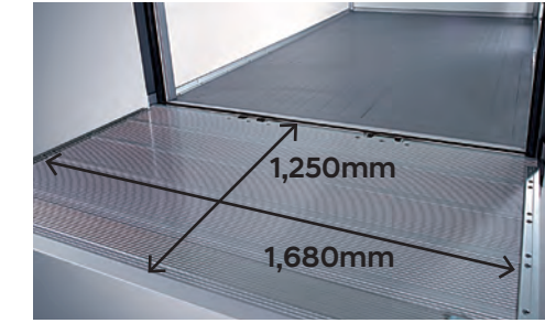
리어도어 겸용 리프트 플레이트
