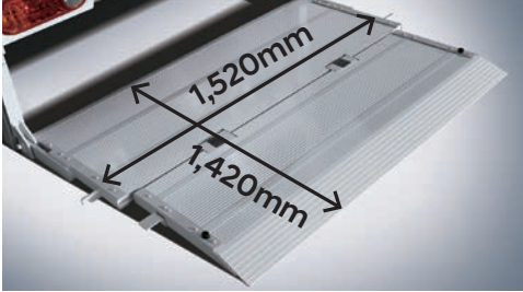
확장형 리프트 패널 (선택)
