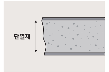
신소재 단열재 ASA시트+ EPS 네오폴 적용(냉동부 측면 65mm)
